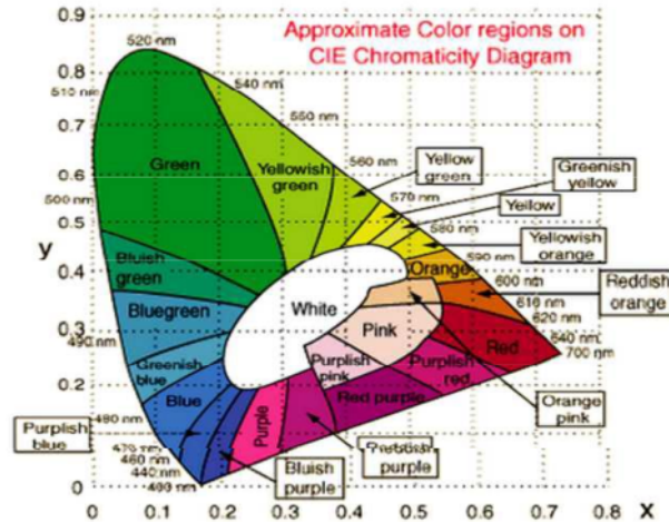
Gambar 3. Diagram Kromatisasi CIE. 4
