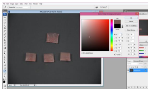
Gambar 5. Hasil CIELab
