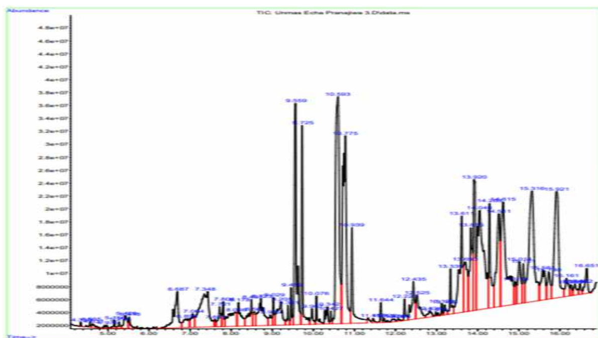
Gambar 1. Grafik kromatogram ekstrak buah tumbuhan purnajiwa
