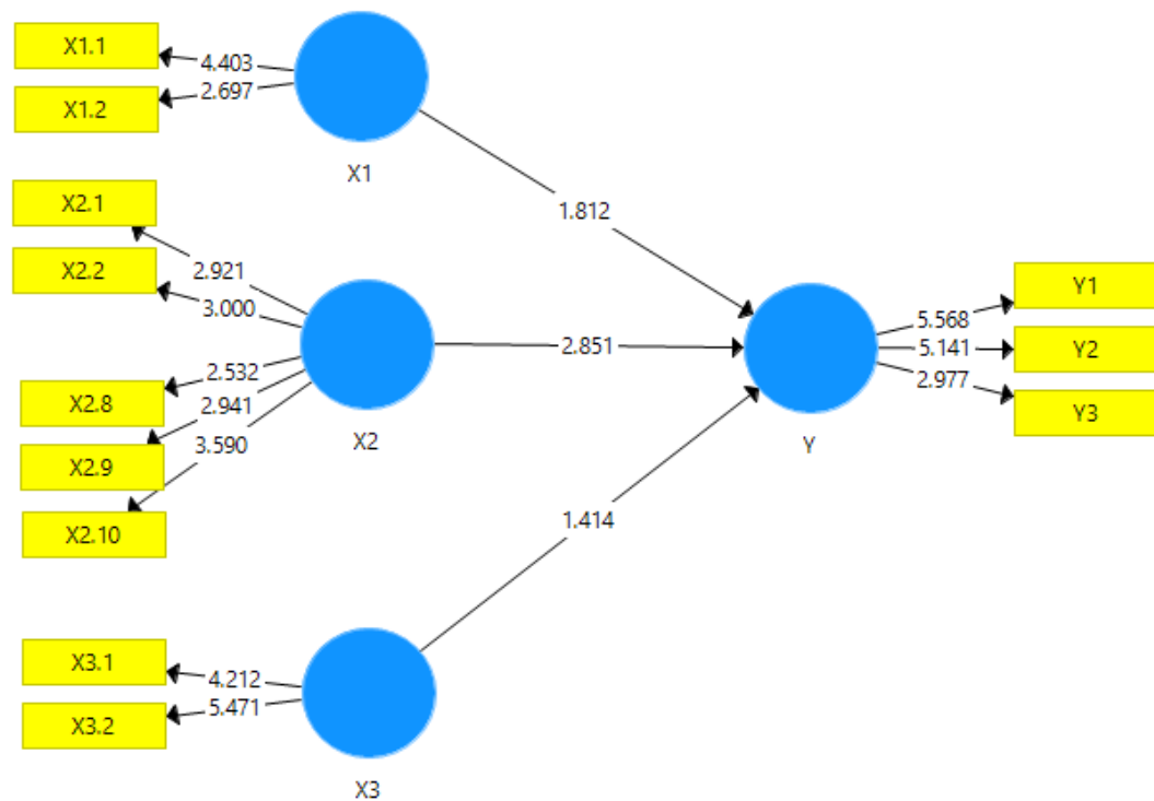
Gambar 3 Pathdiagram setelah bootstraping
