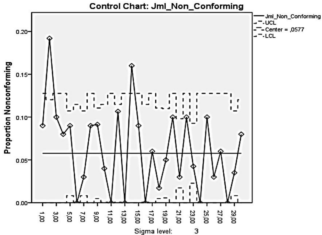
Gambar 2. p-control chart kerusakan produk pada KWT Ayu Tangkas.
