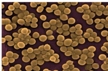
Gambar 1. Bentuk mikroskopis S. aureus
